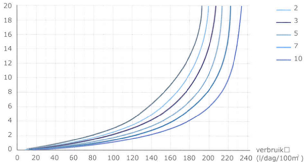
Figuur: Regenwaterdimensioneringsgrafiek
